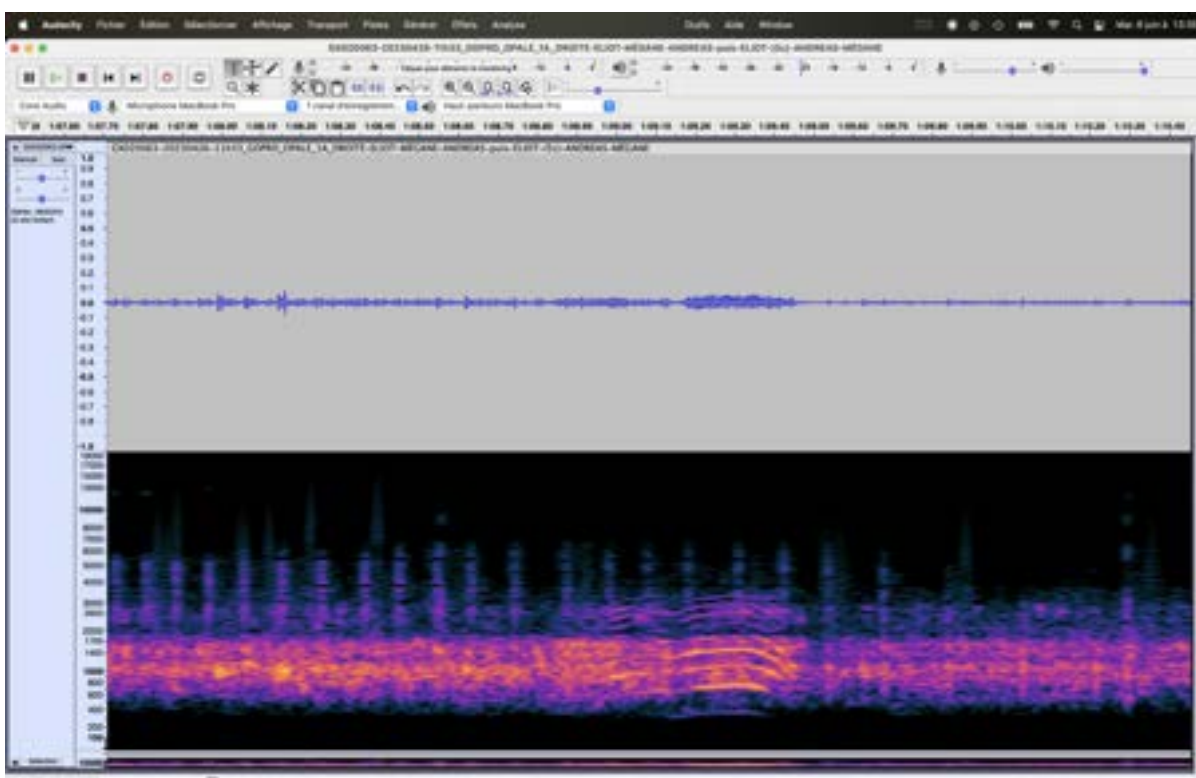
Spectrogramme et forme d'onde du miaulement de Andreas
