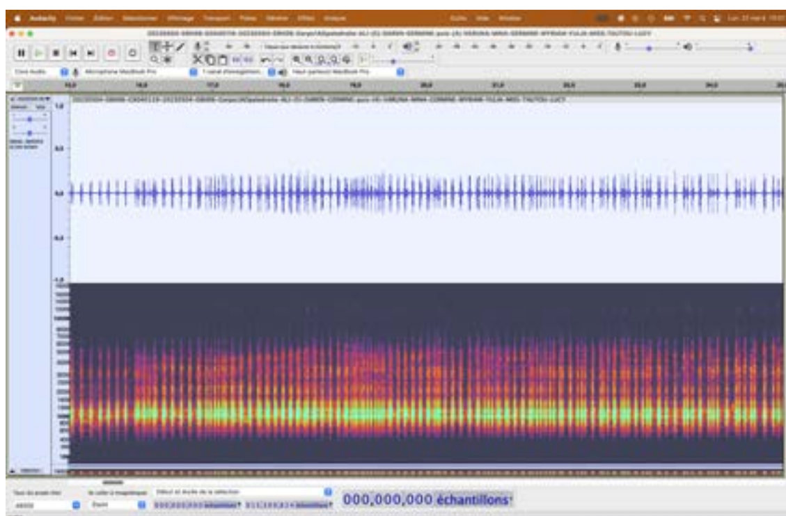
Forme d'onde et spectro des staccatos de clics lors de la confrontation entre Ali et Daren
