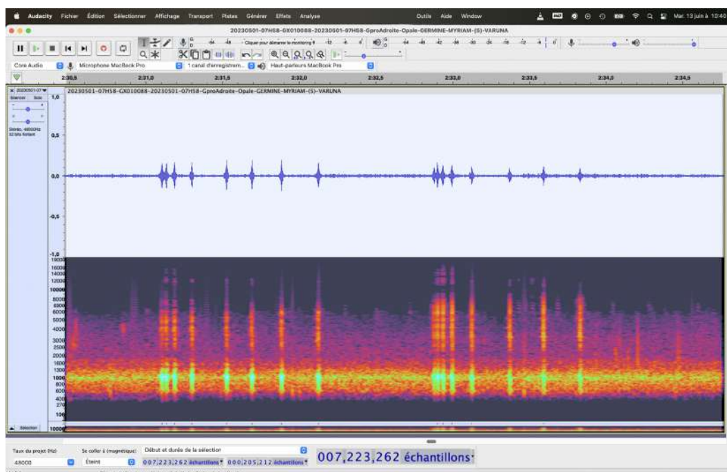
Forme d'onde et spectrogramme des échanges de codas entre Myriam et Varuna
