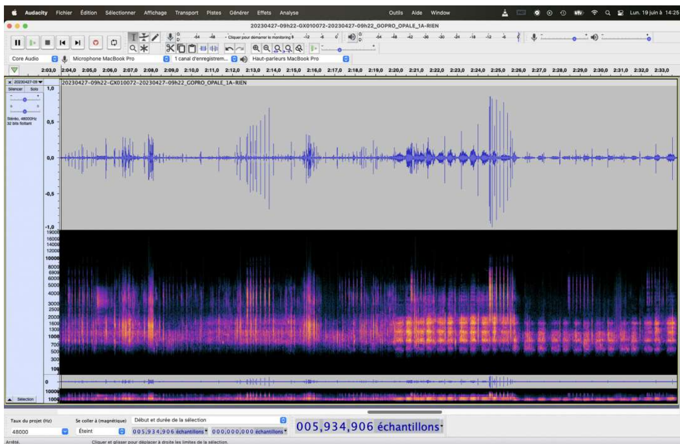
Forme d'onde et spectrogramme avec codas, alors que Delphine semble en relation 5C avec un cachalot non identifié
