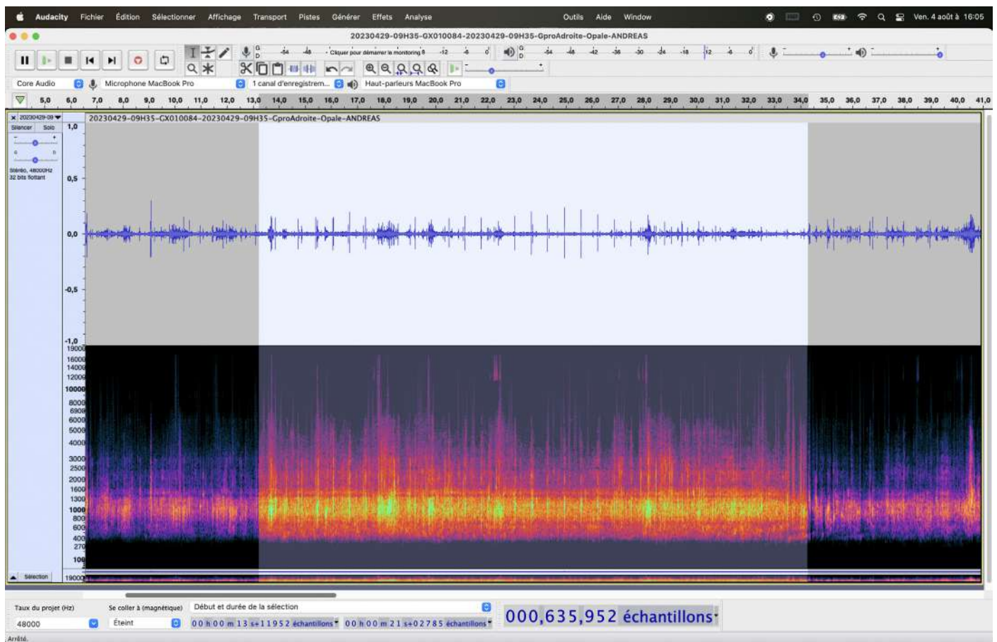
Forme d'onde et spectrogramme des clics de fond émis par les cachalots lors de leurs chasses profondes
