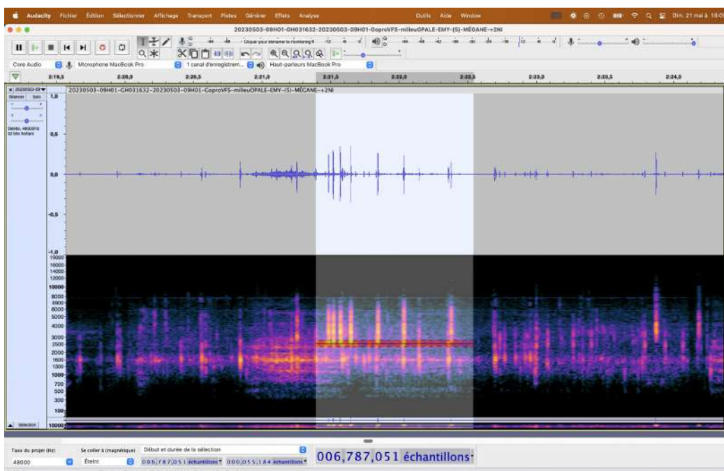
Forme d'onde et spectrogramme de l'échange de codas entre Emy et Mégane
