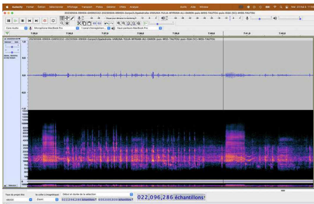
Forme d'onde et spectrogramme de staccatos de clics et d'un miaulement de Myriam
